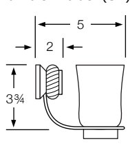
316-0.6 Tumbler Holder (SV)
