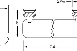
316-0.8 Glass Shelf (TV)
